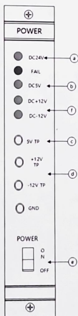
2.13 - сурет – Электрмен қоректендіру модулінің алдыңғы бөлігі сұлбасы
