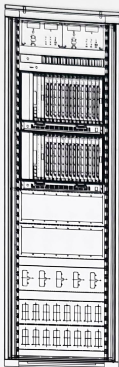
2.6 - сурет – Логикалық орталықтандыру стойкасы – EIER
