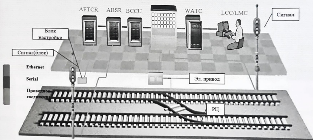
2.4 - сурет – Метрополитендегі электрондық орталықтандыру (EIE) құрылымдық сұлбасы
