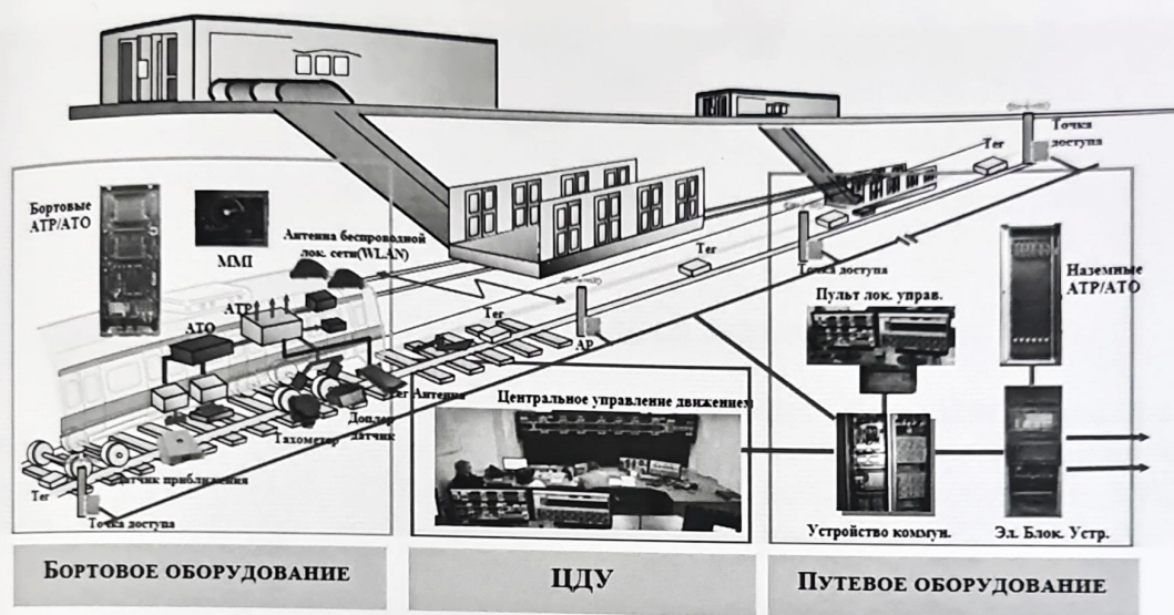
2.2 - сурет – CBTC жүйесінің құрылымдық сұлбасы
