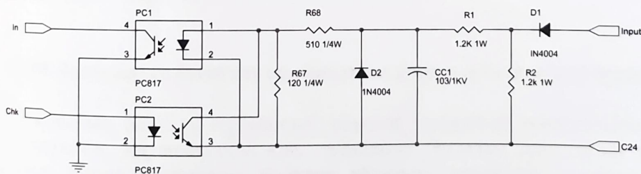
2.17 - сурет – Деректерді енгізу блогының электрлік сұлбасы
