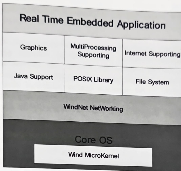
2.11 - сурет – Бағдарламалық қамсыздандырудың негізгі құрылымы
