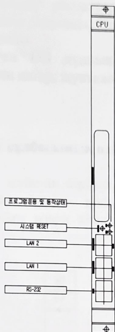
2.14 - сурет – Модуль құрылымының алдыңғы бөлігінің сұлбасы
