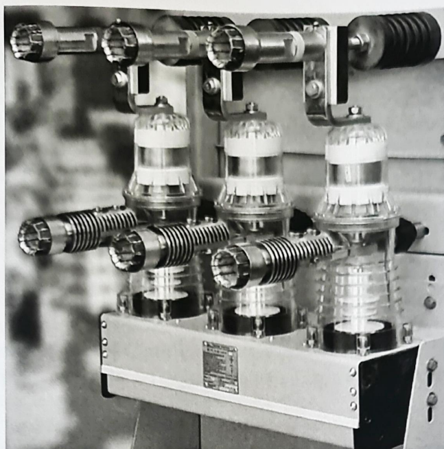
3.1 - сурет – BB/TEL ажыратқышының бейнесі
