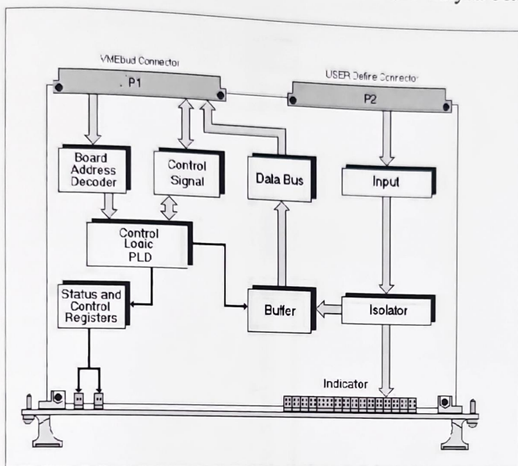
2.18 - сурет – Деректерді енгізу модулінің блоктар сұлбасы
